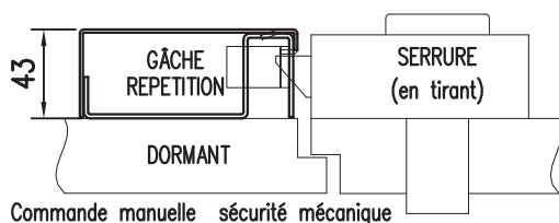
Gâche Répétition Tirant
