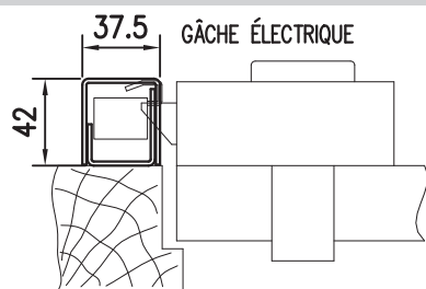
Gâche en Applique électrique
