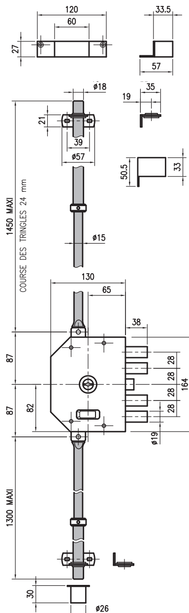
SERRURE CR
